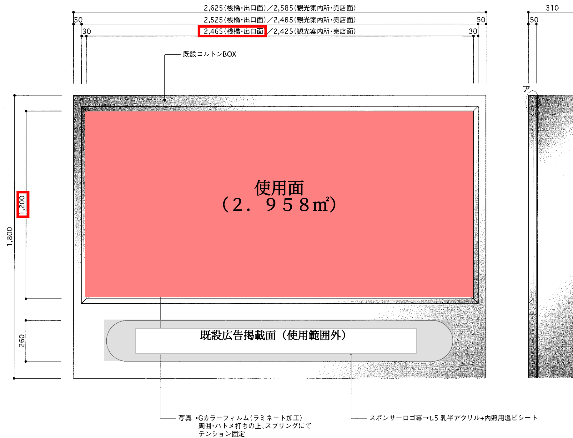
正面図 S:1/10
