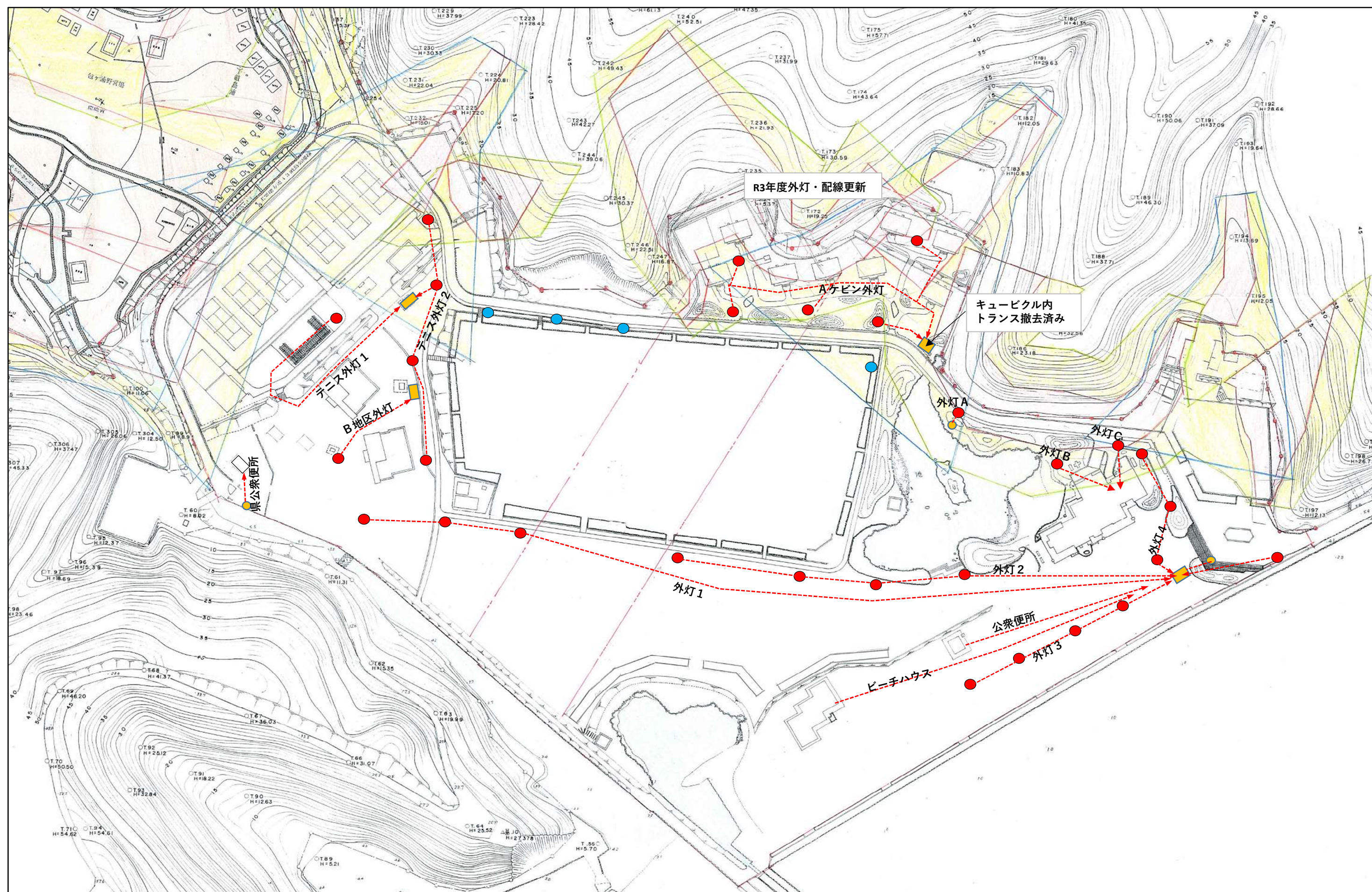
外灯配置図（グラウンド周辺）
