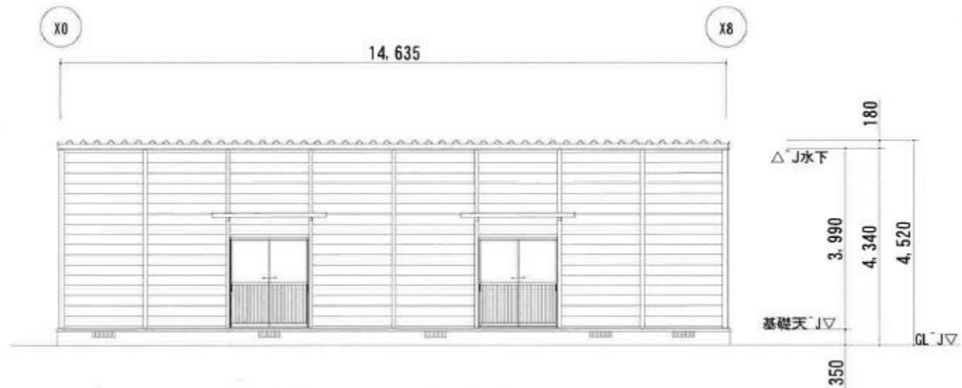
Y2 立面図 S=1/100
