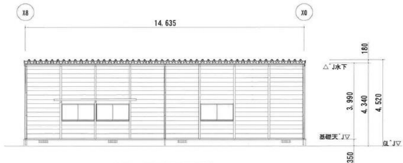
Y0 立面図 S=1/100
