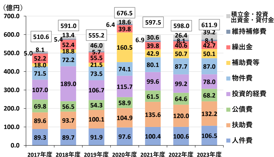
図 2-49 歳出の推移
