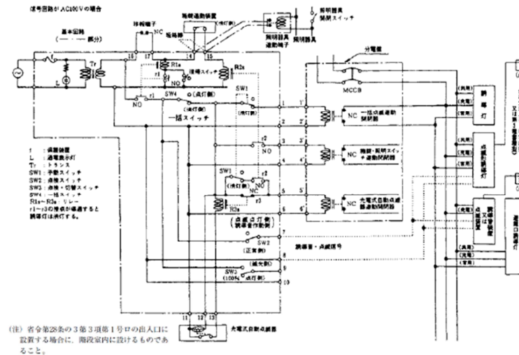
図16-22 機器結線図
