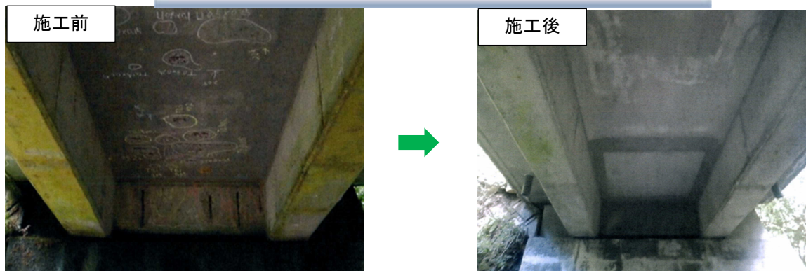
橋りょうの長寿命化工事の例（阿品台中央橋）
