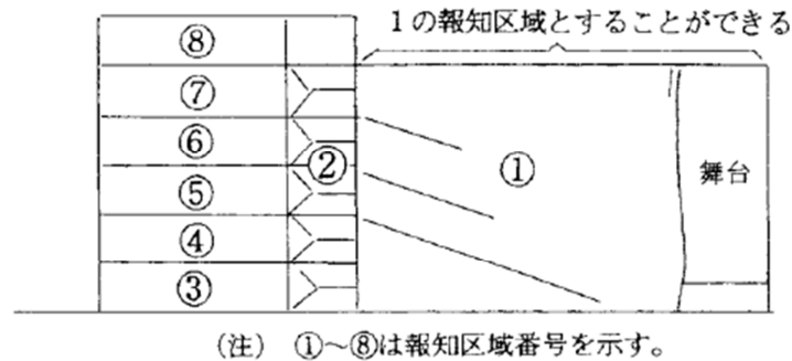
図14—1 吹き抜けがある場合の報知区域の設定例
