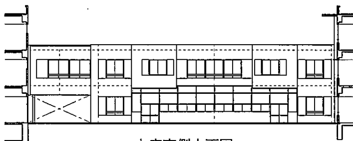
中庭南側立面图
