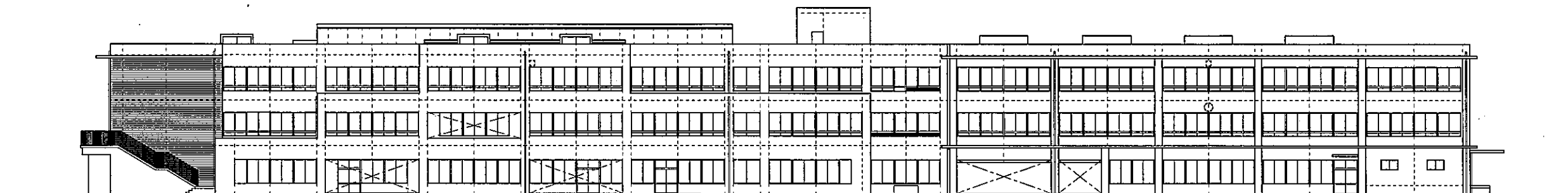
北側立面图
