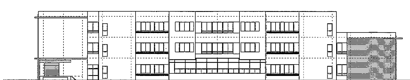
西側立面图
