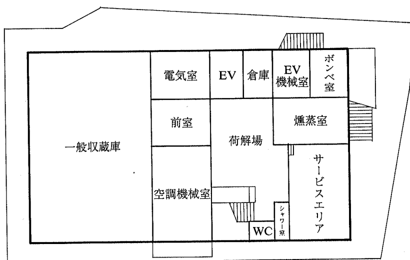
地階平面図
