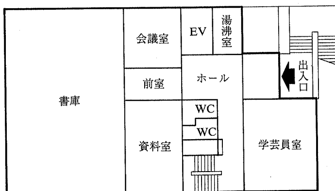
1 階平面図
