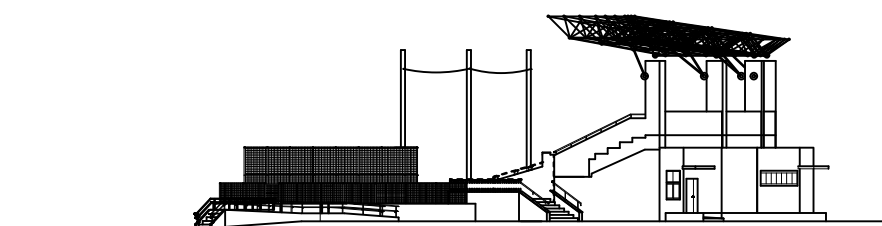
東側立面図
