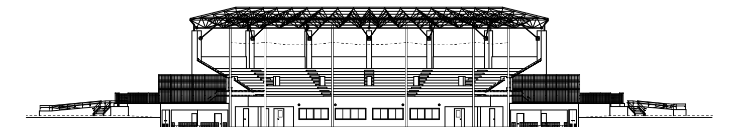
南側(グランド側)立面図
