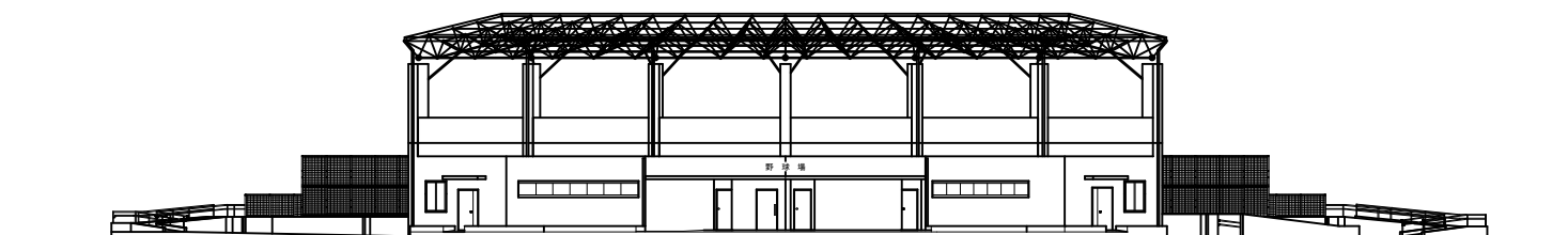
北側立面図
