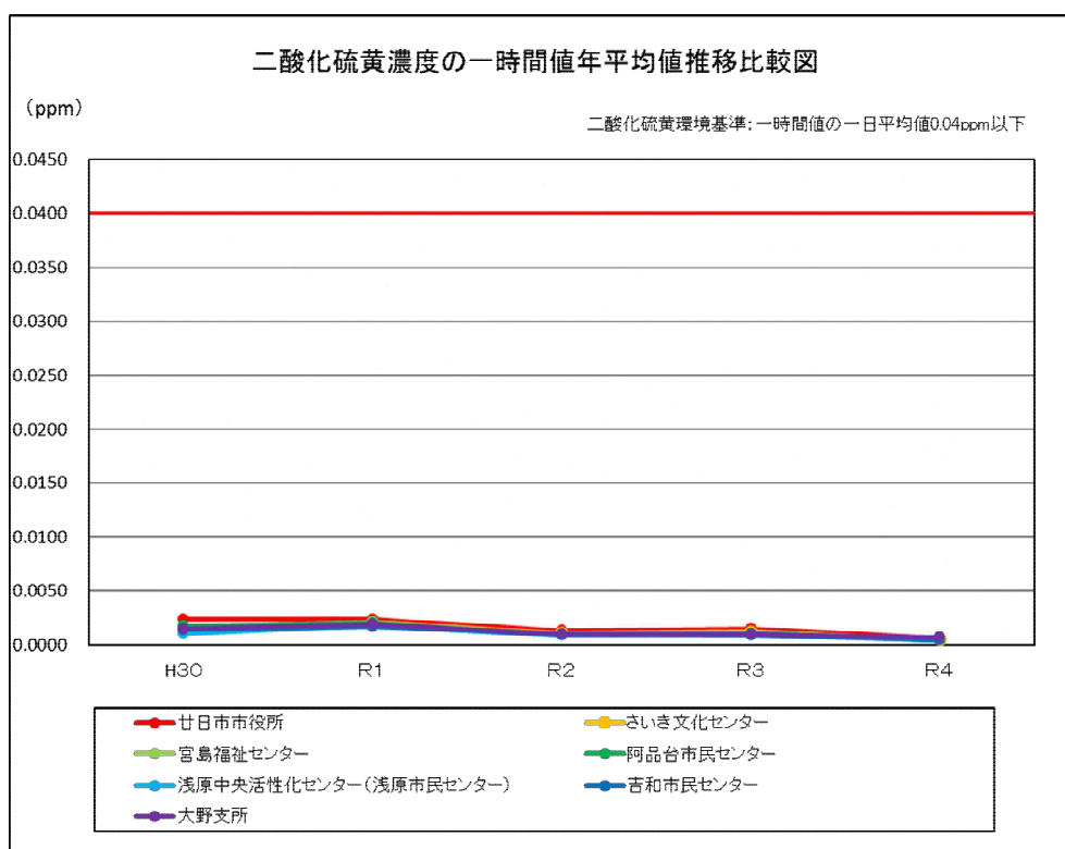
(図Ⅳ－４) 二酸化硫黄濃度の一時間値年平均値推移比較図
