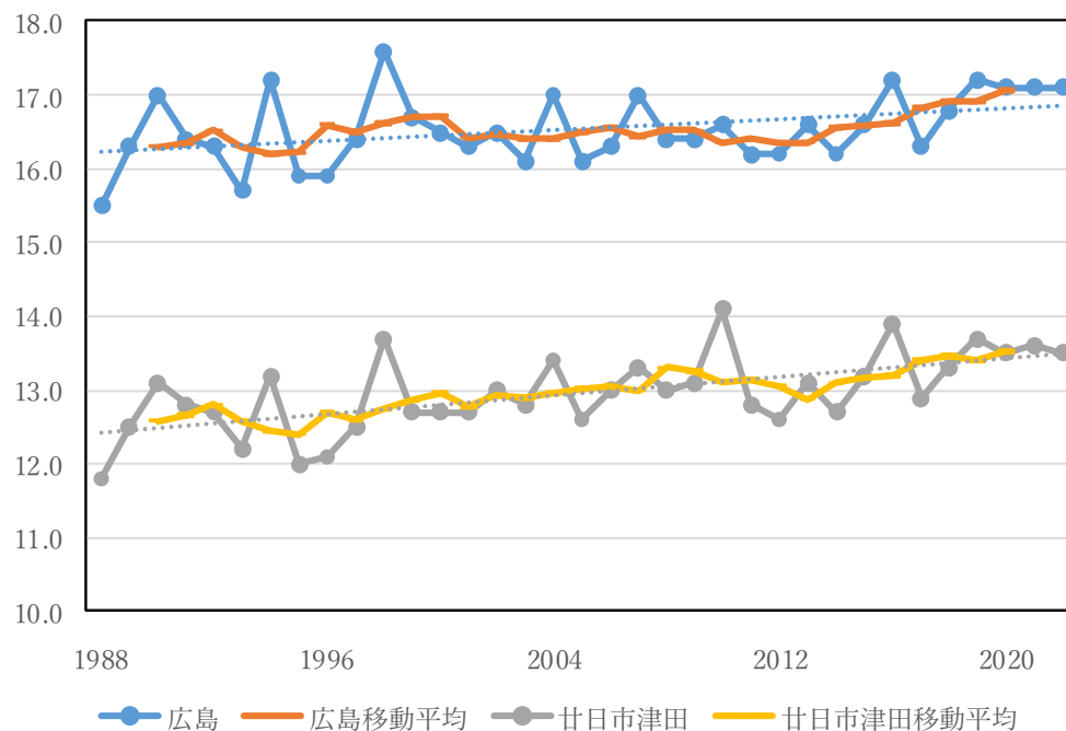
（図IX-4） 広島及び廿日市津田における年平均気温の推移
