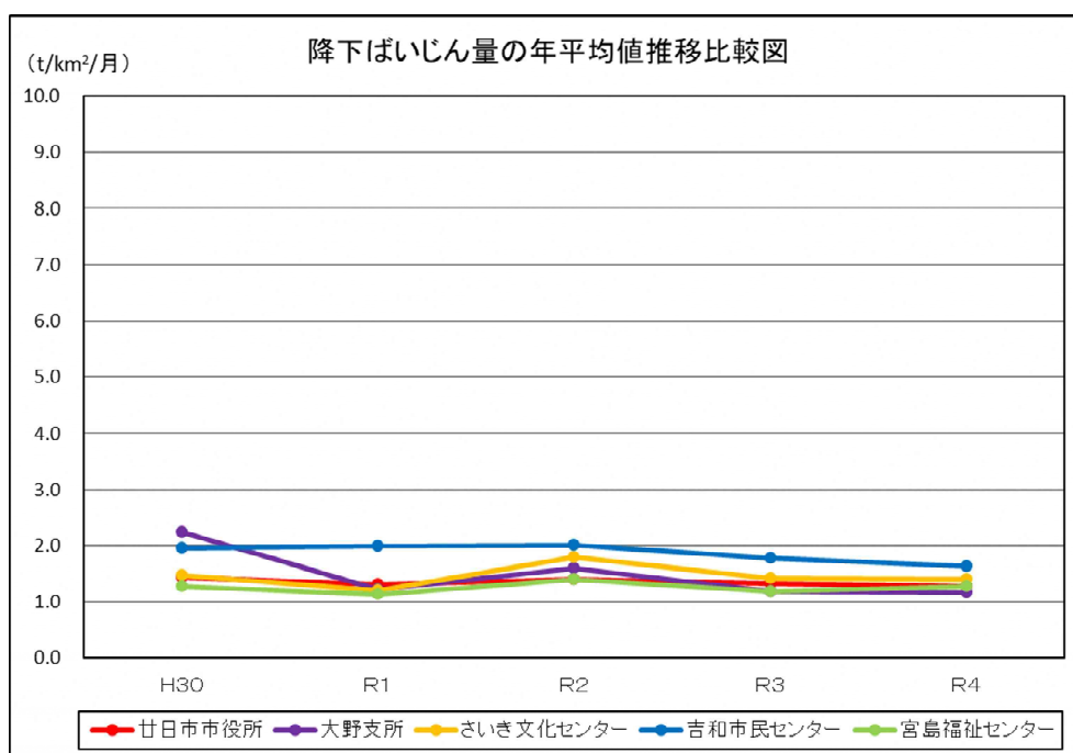
(図IV－7) 降下ばいじん量の年平均値推移比較図
