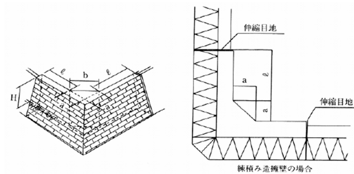
(a) 立体図
