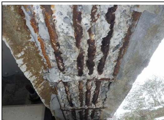
主桁の腐食(コンクリート桁)
