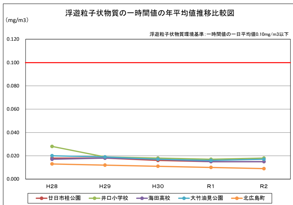
(図IV－6) 浮遊粒子状物質の一時間値の年平均値推移比較図
