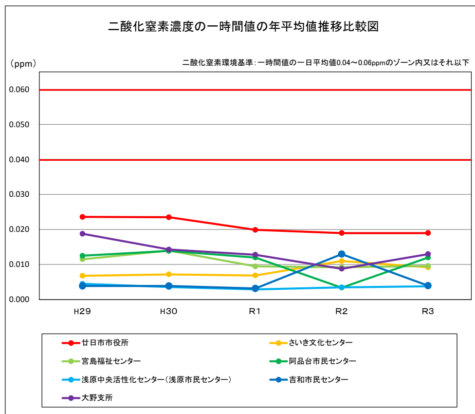
(図Ⅳ－５) 二酸化窒素濃度の１時間値の年平均値推移比較図
