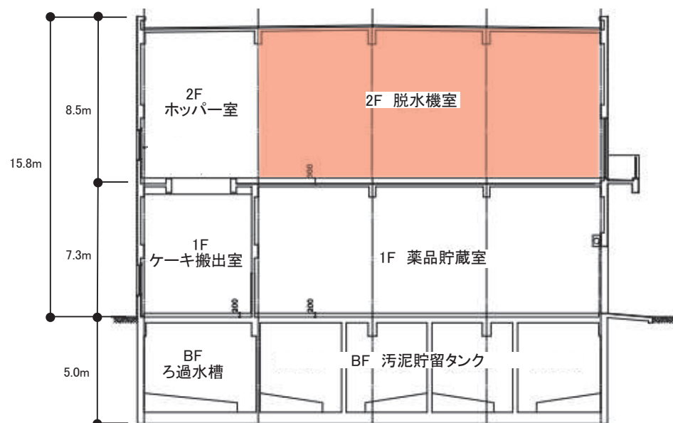
断面図(南側)
