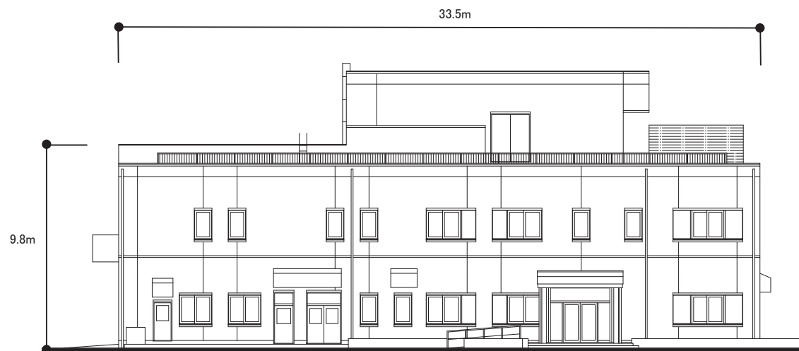
立面図(南)
