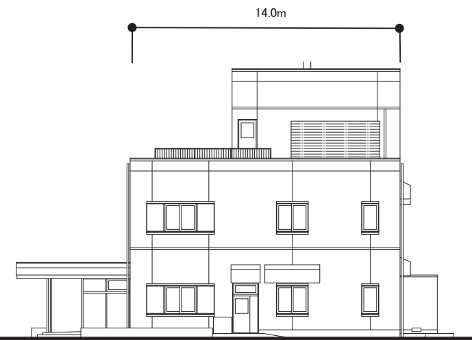
立面図(東)
