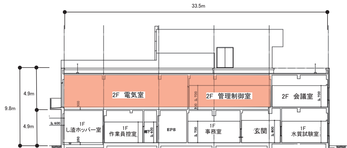
断面図(南側)
