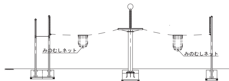
カーカ断面図
