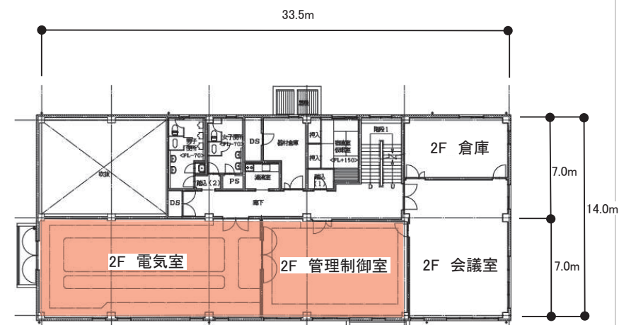
平面図(2階)
