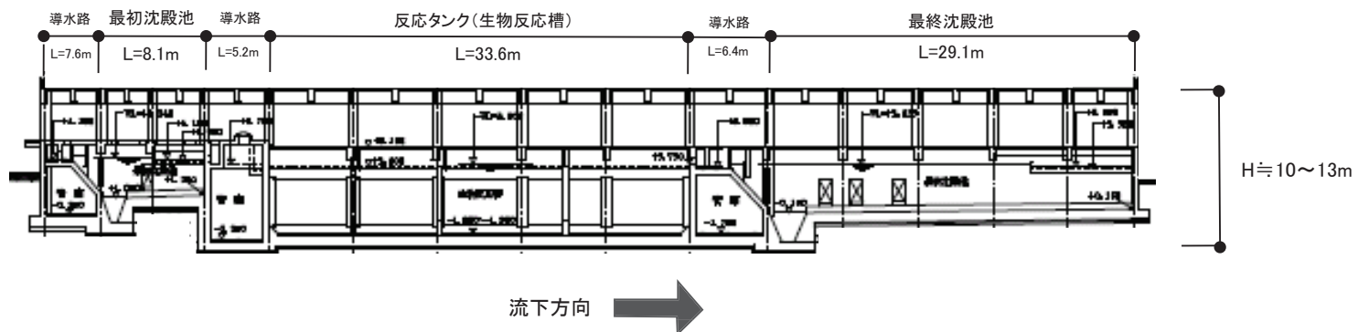
断面図
