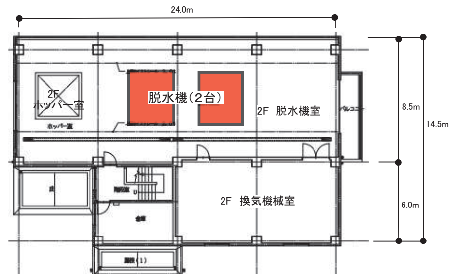
平面図(2階)
