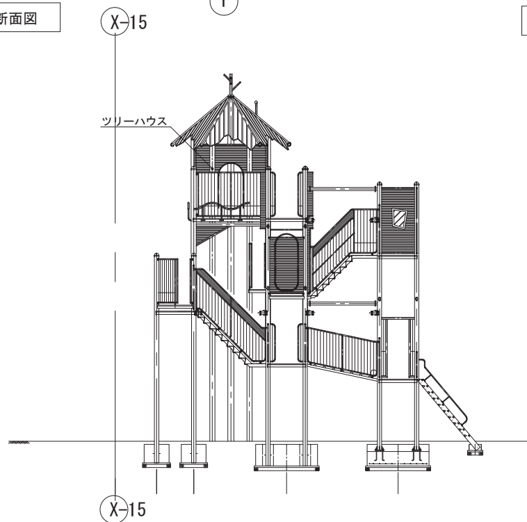
ウーウ断面図
