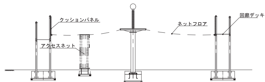
カーカ断面図
