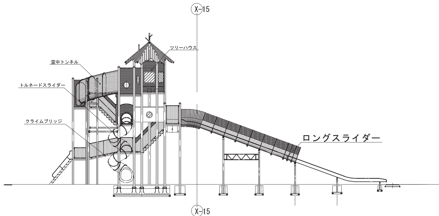
エーエ断面図
